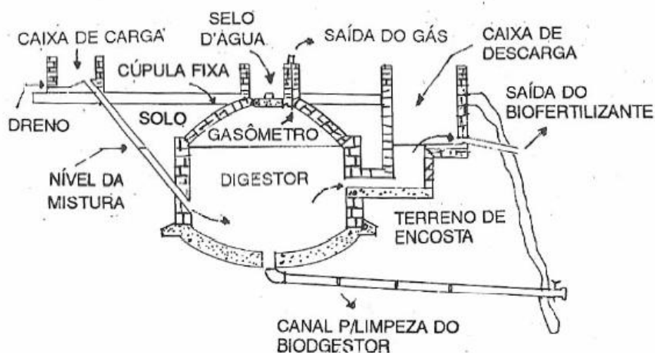
Figura 6 - Biodigestor modelo chinês.
