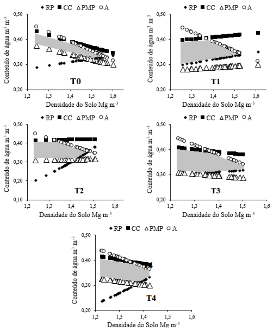
Figura 9. IHO, conteúdo de água na capacidade de campo ( \theta_{CC} ), ponto de murcha permanente ( \theta_{PMP} ), porosidade de aeração de 0,10 \text{ m}^3 \text{m}^{-3} ( \theta_{PA} ) e resistência do solo a penetração de 2,0 \text{ MPa} ( \theta_{RP} ), em função da densidade de um Latossolo Vermelho distroférrico, sob colheita mecanizada de cana-de-açúcar submetidos a diferentes níveis de palhicho no solo, na profundidade de 0,30 \text{ m} . “T0” Sem palhicho; “T1” 5 \text{ Mg ha}^{-1} ; “T2” 10 \text{ Mg ha}^{-1} ; “T3” 15 \text{ Mg ha}^{-1} e “T4” 20 \text{ Mg ha}^{-1} .
