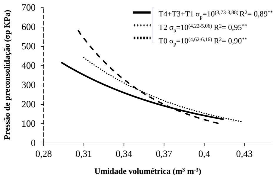
Figura 10. Modelos de capacidade de suporte de carga para um Latossolo Vermelho distroférico, sob colheita mecanizada de cana-de-açúcar submetidos a diferentes níveis de palhicho no solo, na profundidade 0,10 m. T0” Sem palhicho; “T1” 5 Mg ha -1 ; “T2” 10 Mg ha -1 ; “T3” 15 Mg ha -1 e “T4” 20 Mg ha -1 .
